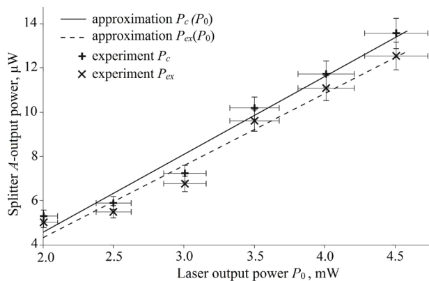
Рисунок 4 – Измеренные мощности циркуляции P_c и мощности вывода P_{ex} в зависимости от выходной мощности лазерного источника P_0
