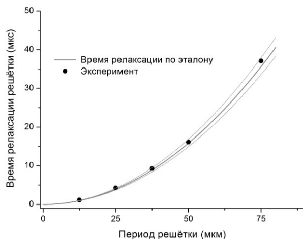
Рисунок 2 – Сопоставление измеренного времени релаксации тепловой решетки в рабочем эталоне из нержавеющей стали 12X18H10T (ГОСТ 5632-72) с номинальным временем релаксации, рассчитанным из паспортного значения температуропроводности
