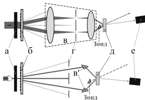
Рисунок 1 – Оптическая схема комплекса «Оптопикотест»: а – аттенюатор; б – светоделитель; в – телескоп; в' – поворотные призмы; г – пространственный фильтр; д – образец; е – фотоприемник
