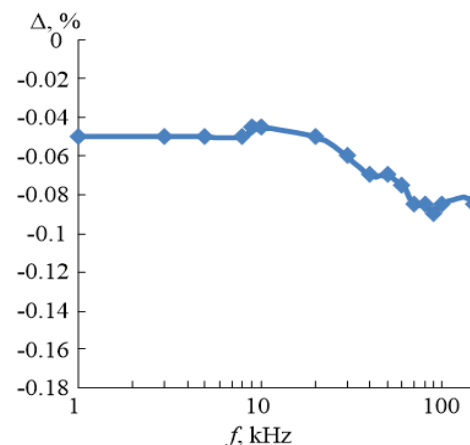
Рисунок 3 – Зависимость погрешности преобразования синусоидального сигнала с V_{OUTRMS} = 1 В от частоты для преобразователя переменного напряжения без усилителя
